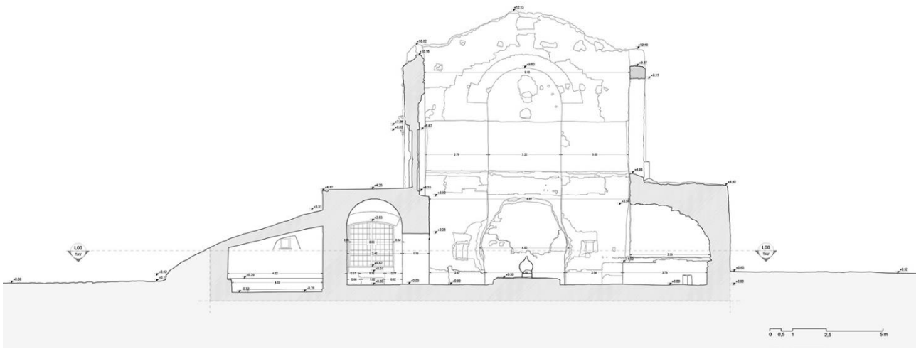
Sezione longitudinale BB del mausoleo.
