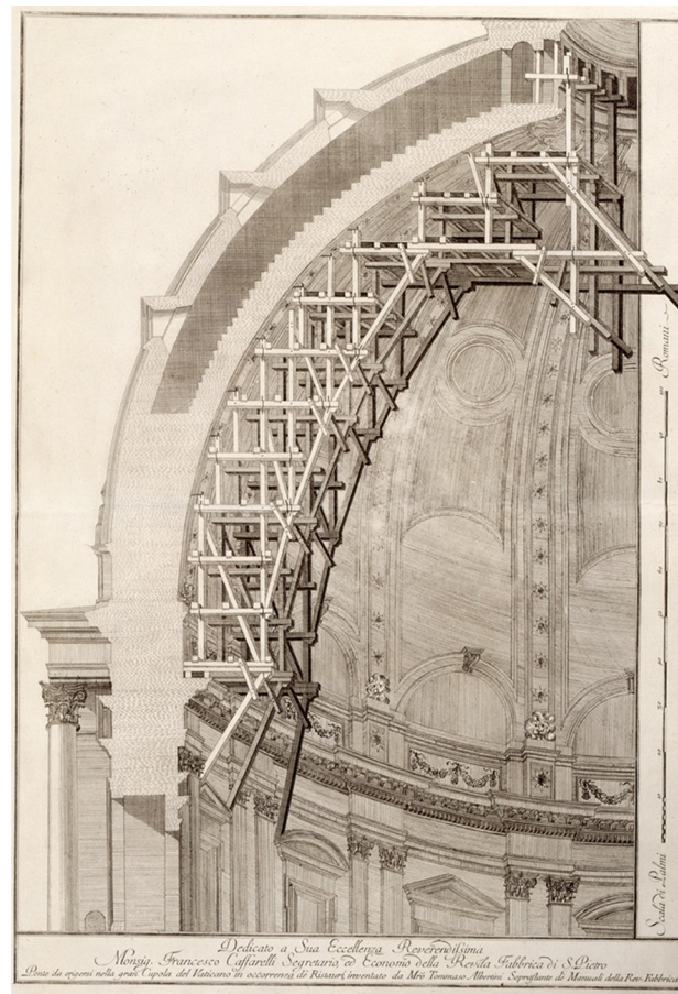
Tommaso Albertini, Ponte da erigersi nella gran Cupola del Vaticano in occasione de' Ristauri, in Castelli e ponti di Nicola Zabaglia, Roma 1824, tav. LVII.
